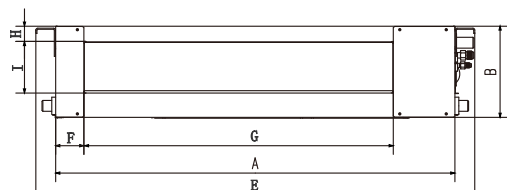
Tamanho da abertura de retorno de ar (retorno por trás):
