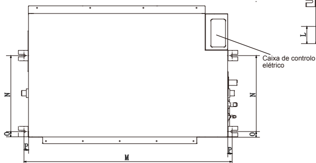
Distância entre os anéis de suspensão
